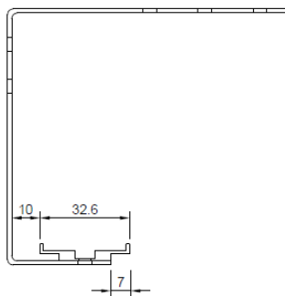
ダブルレール(LOR-TLD)装着イメージ
