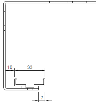
ダブルレール(LOR-IPD)装着イメージ
