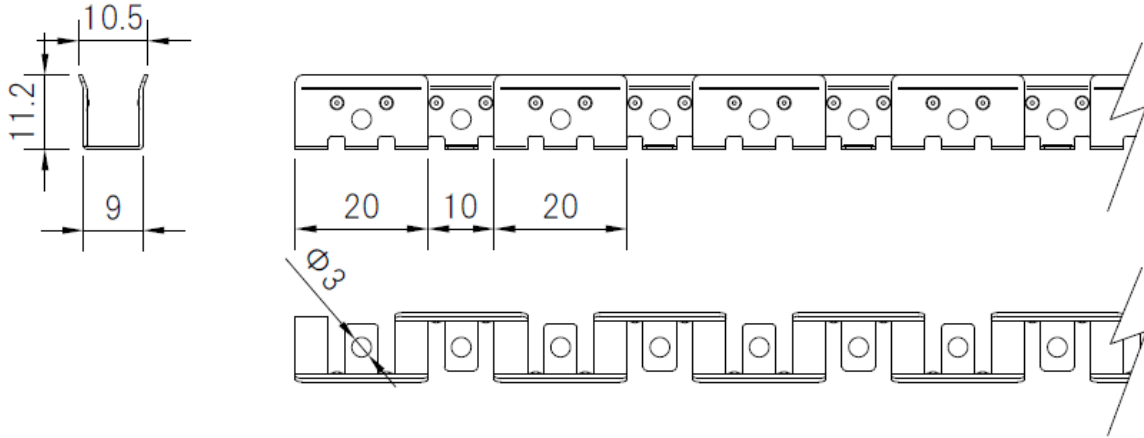
第三角法 (単位mm)
