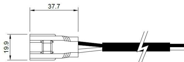
オス側コネクタ
