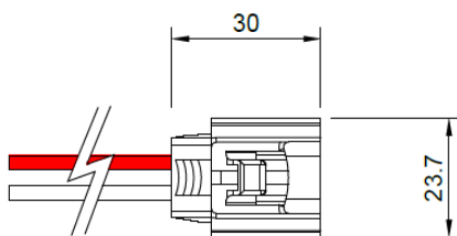
メス側コネクタ-
