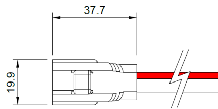
オス側コネクタ-
