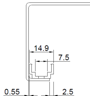
シングルレール(LOR-IPS)装着イメージ
