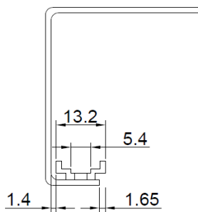
シングルレール(LOR-TLS)装着イメージ
