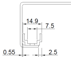
シングルレール(LOR-IPS)装着イメージ
